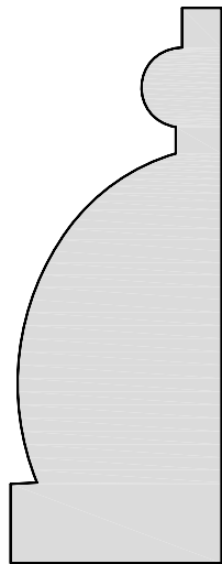
5961 1" x 2 5/8"
